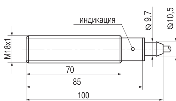
Габаритный чертеж
