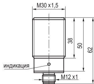
Габаритный чертеж
