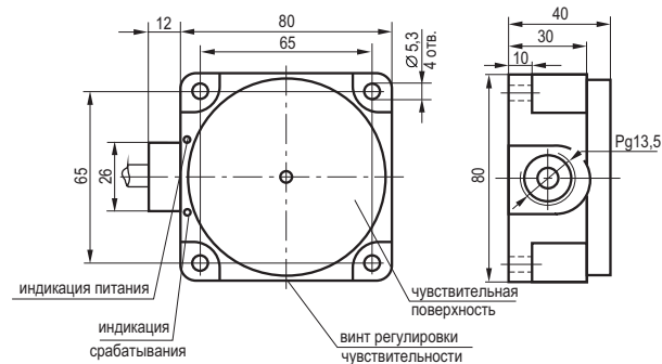
Габаритный чертеж
