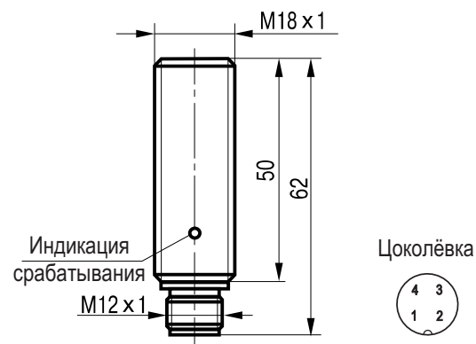
Габаритный чертеж.
