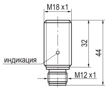
Габаритный чертеж
