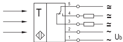
Схема подключения
