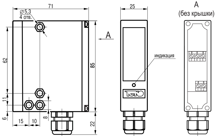
Габаритный чертеж.
