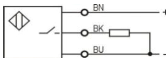
PNP NO
