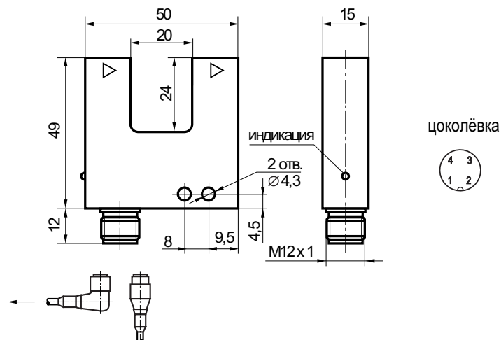
Габаритный чертеж
