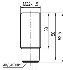
Габаритный чертеж
