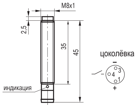
Габаритный чертеж
