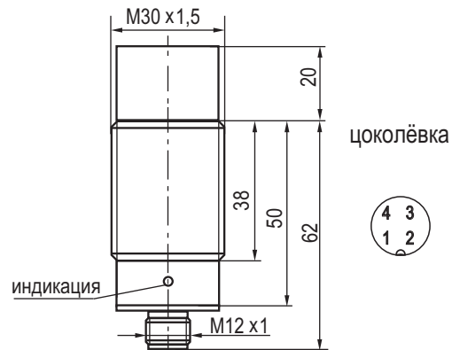
Габаритный чертеж
