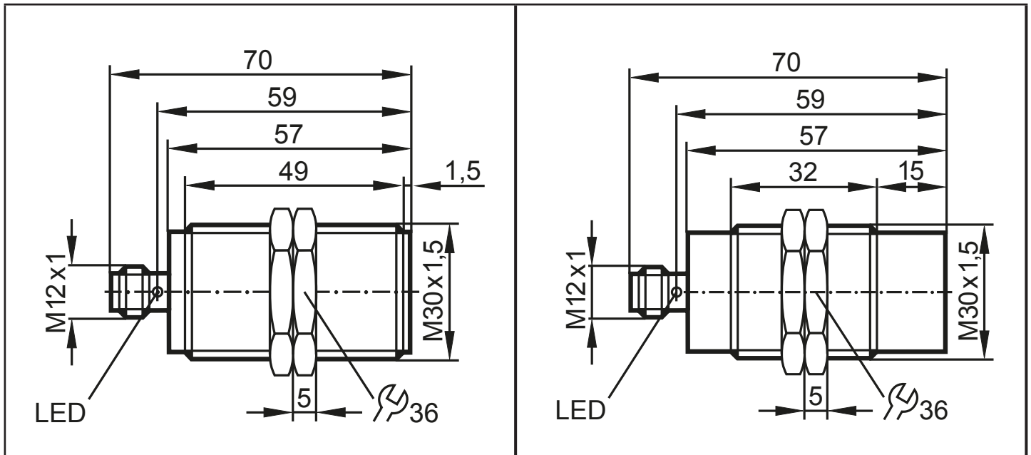
DTM434 / DTM436
