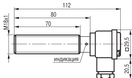
Габаритный чертеж
