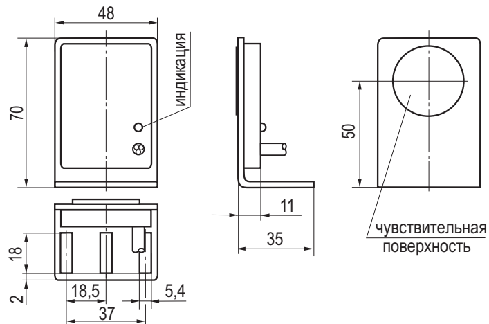
Габаритный чертеж
