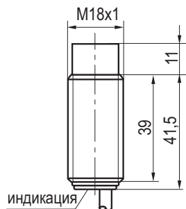
Габаритный чертеж
