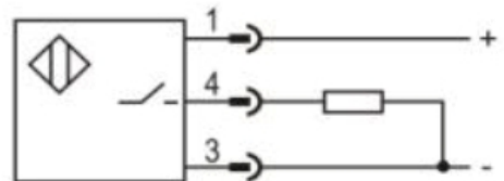
PNP NO
