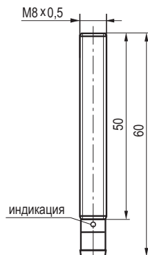
Габаритный чертеж
