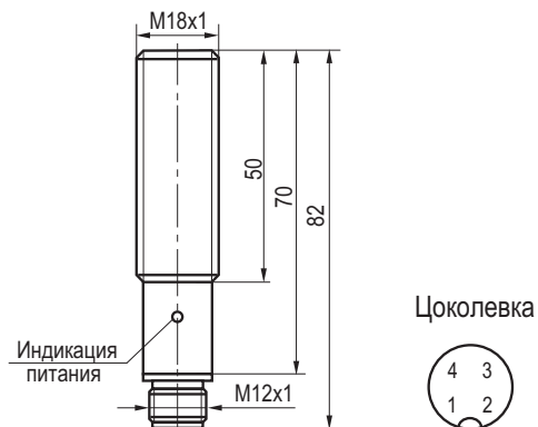
Габаритный чертеж
