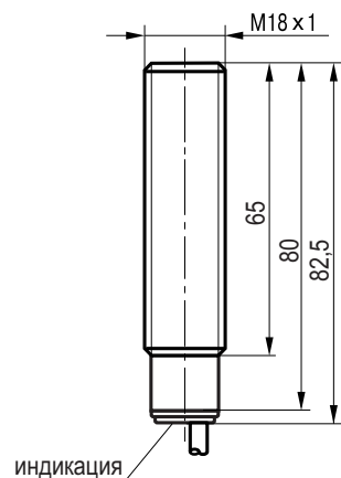
Габаритный чертеж.
