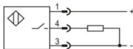
PNP NO
