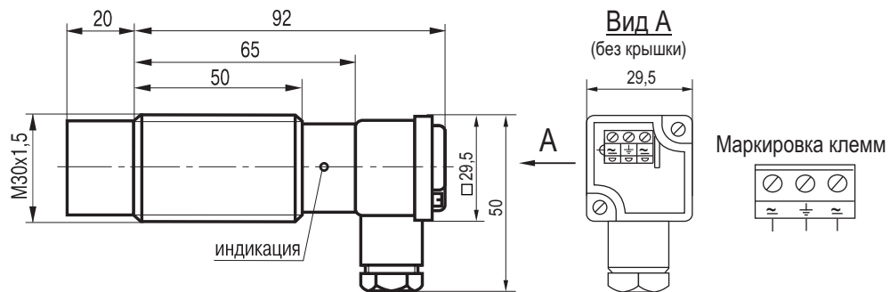
Габаритный чертеж
