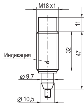
Габаритный чертеж
