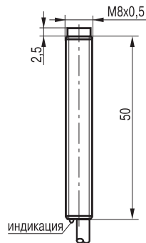
Габаритный чертеж
