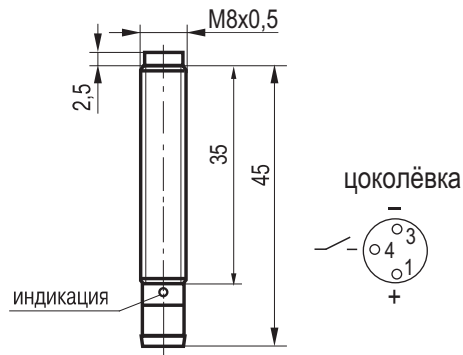
Габаритный чертеж
