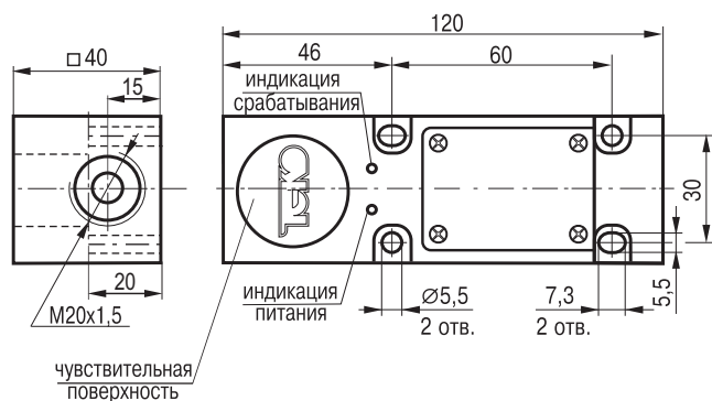
Габаритный чертеж
