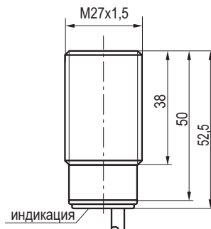
Габаритный чертеж
