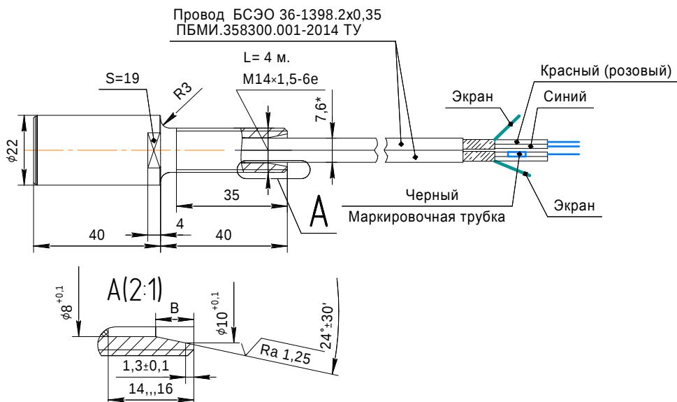
Рисунок 1. Схема подключения ВТИЮ.1467
