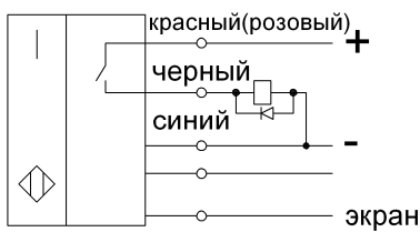
Схема подключения индуктивной нагрузки
