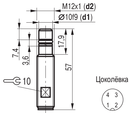
Схема монтажа
