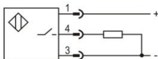
PNP NO
