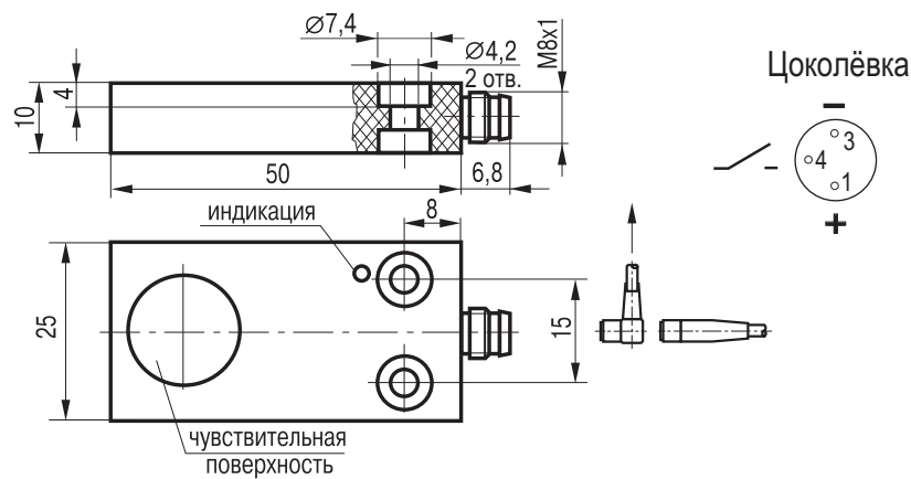
Габаритный чертеж
