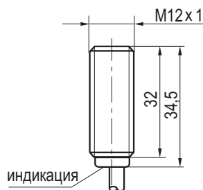
Габаритный чертеж
