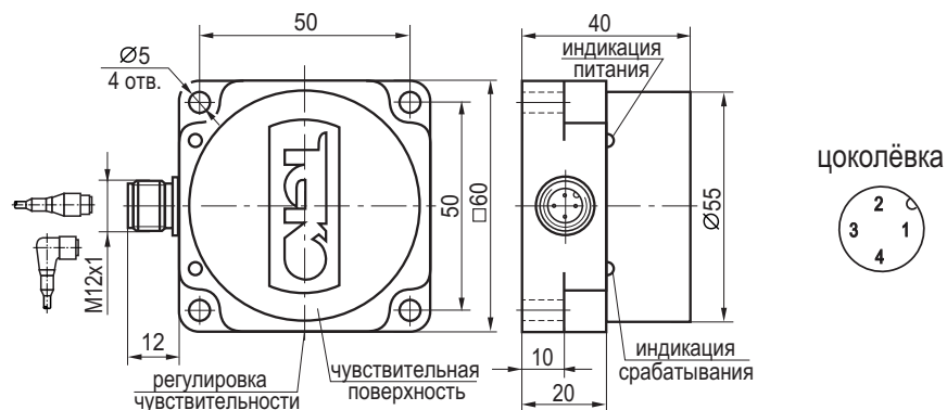
Габаритный чертеж
