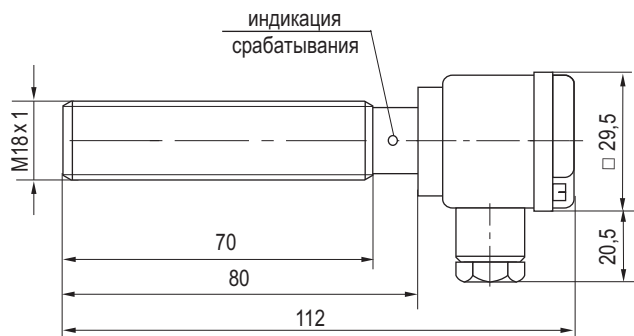
Габаритный чертеж.
