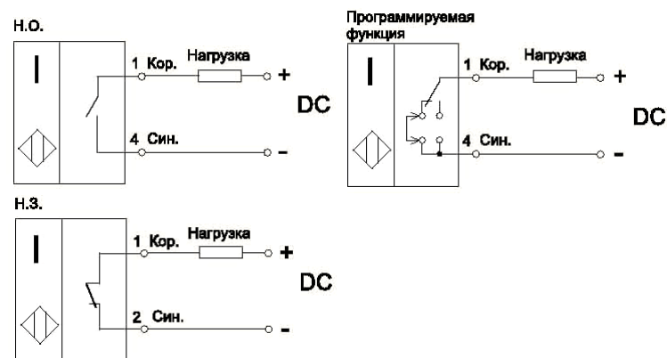
Рис.1. Варианты схем подключения датчиков
