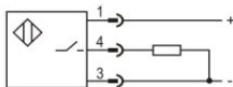
PNP NO
