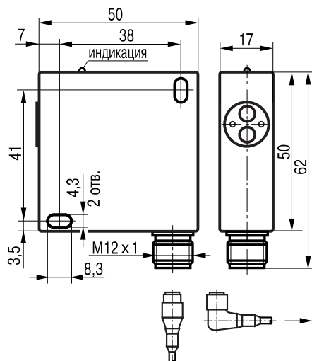
Габаритный чертеж
