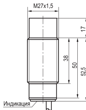
Габаритный чертеж
