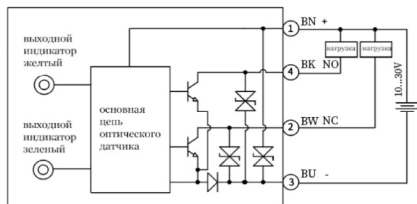
приемник NPN
