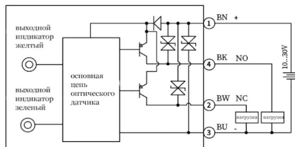
приемник PNP
