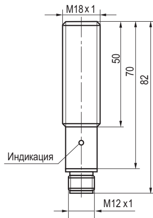
Габаритный чертеж
