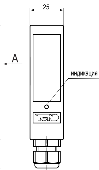
Габаритный чертеж
