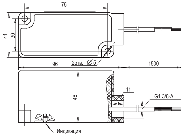
Габаритный чертеж
