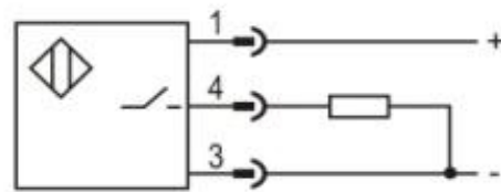
PNP NO
