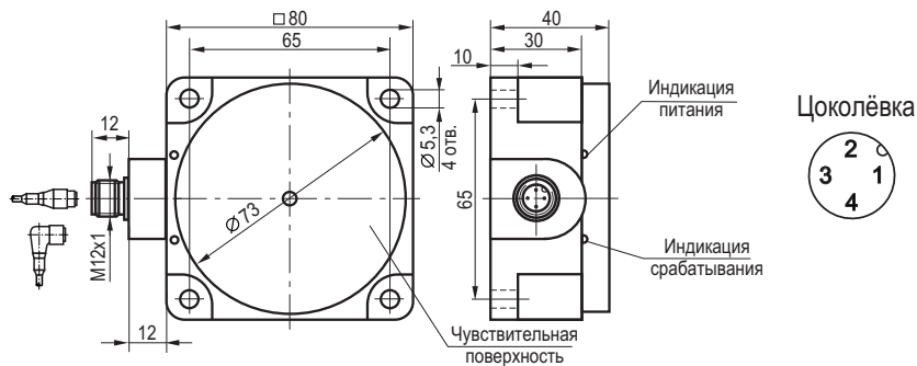
Габаритный чертеж
