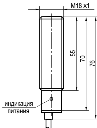
Габаритный чертеж
