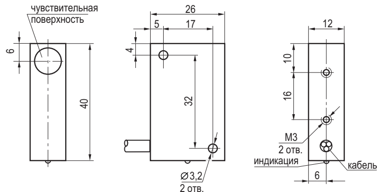
Габаритный чертеж
