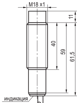
Габаритный чертеж
