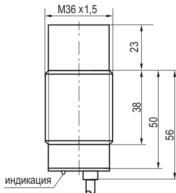
Габаритный чертеж
