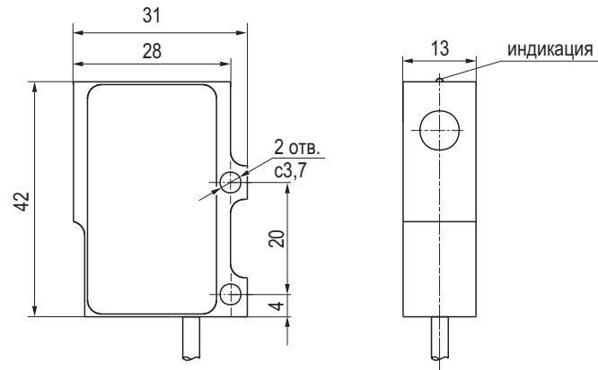
Габаритный чертеж
