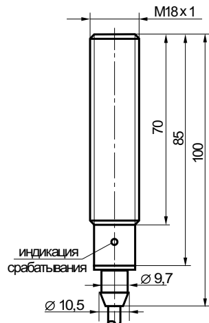
Габаритный чертеж.
