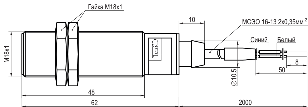
Габаритный чертеж
